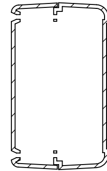
SECCIÓN B-B
