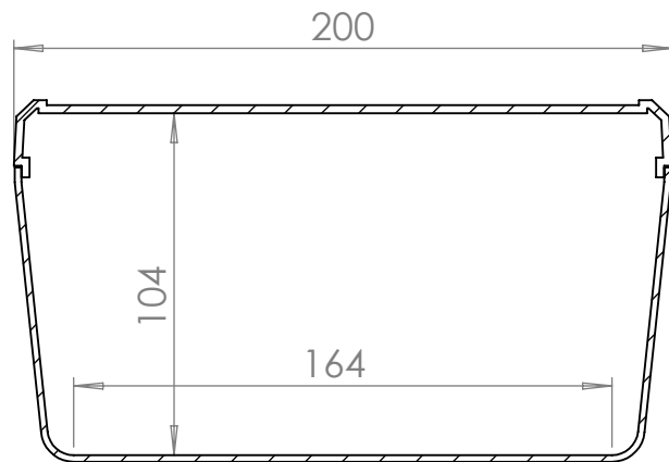
SECCIÓN A-A
