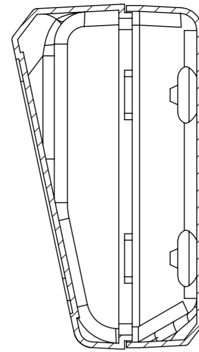
SECCIÓN B-B
