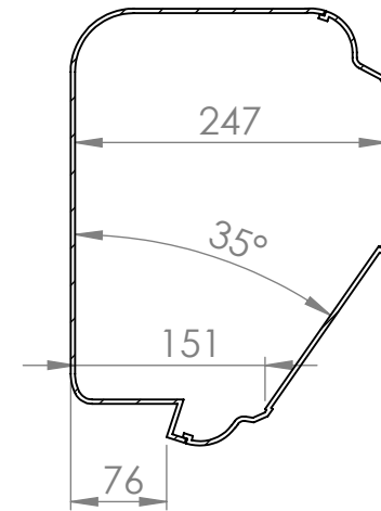
SECCIÓN A-A
