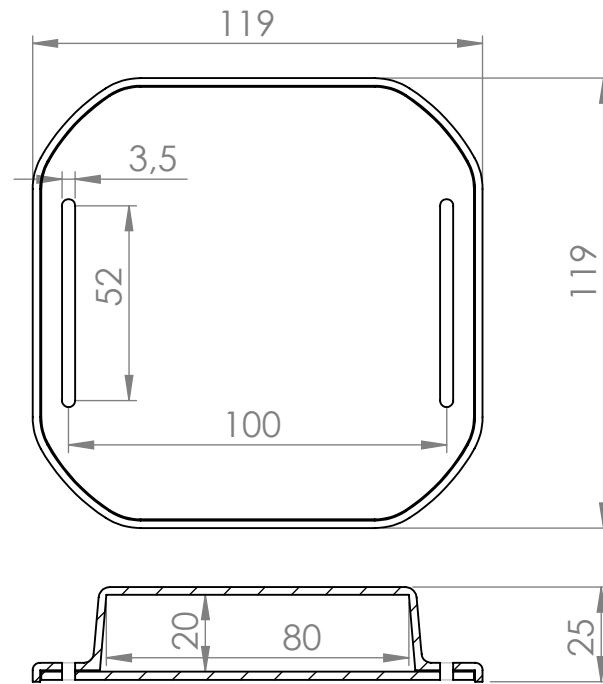
SECCIÓN A-A
