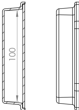
SECCIÓN B-B
